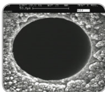
Einspritzöffnung mit DK Premium nach Langzeittest
