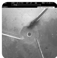
Tangentialslitze der Düse in Makroaufnahme ohne Clean up
