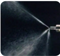
Sprühbild einer verkokten Düse
